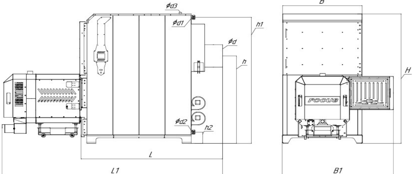
Габаритні розміри пеллетного котла FOCUS PROM
