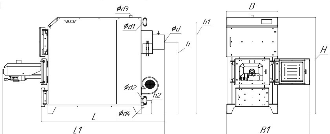
Габаритні розміри пеллетного котла FOCUS
